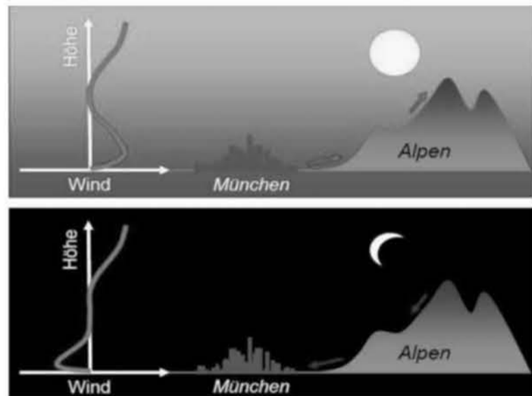
Alpines Pumpen: Tagsüber weht der Wind in Richtung Alpen, nachts weht kühle Luft aus den Alpen in Richtung Stadt. Das alpine Pumpen hat einen erheblichen Einfluss auf das Klima von München und trägt sowohl nachts als auch tagsüber zur Abkühlung bei. (Foto: BI Frischluftzufuhr München)
